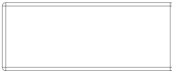
(1) J1 - SOPORTE DE MOSTRADOR - W4L04753 1"x2 3/8"x5 7/8" (24x60x150)
