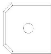
J7 SOPORTE DE VARILLA DE CORTINA EXTERIOR - W4L17101 (x2) 15/16"x2 3/8"x 2 3/8" (24x60x60)
