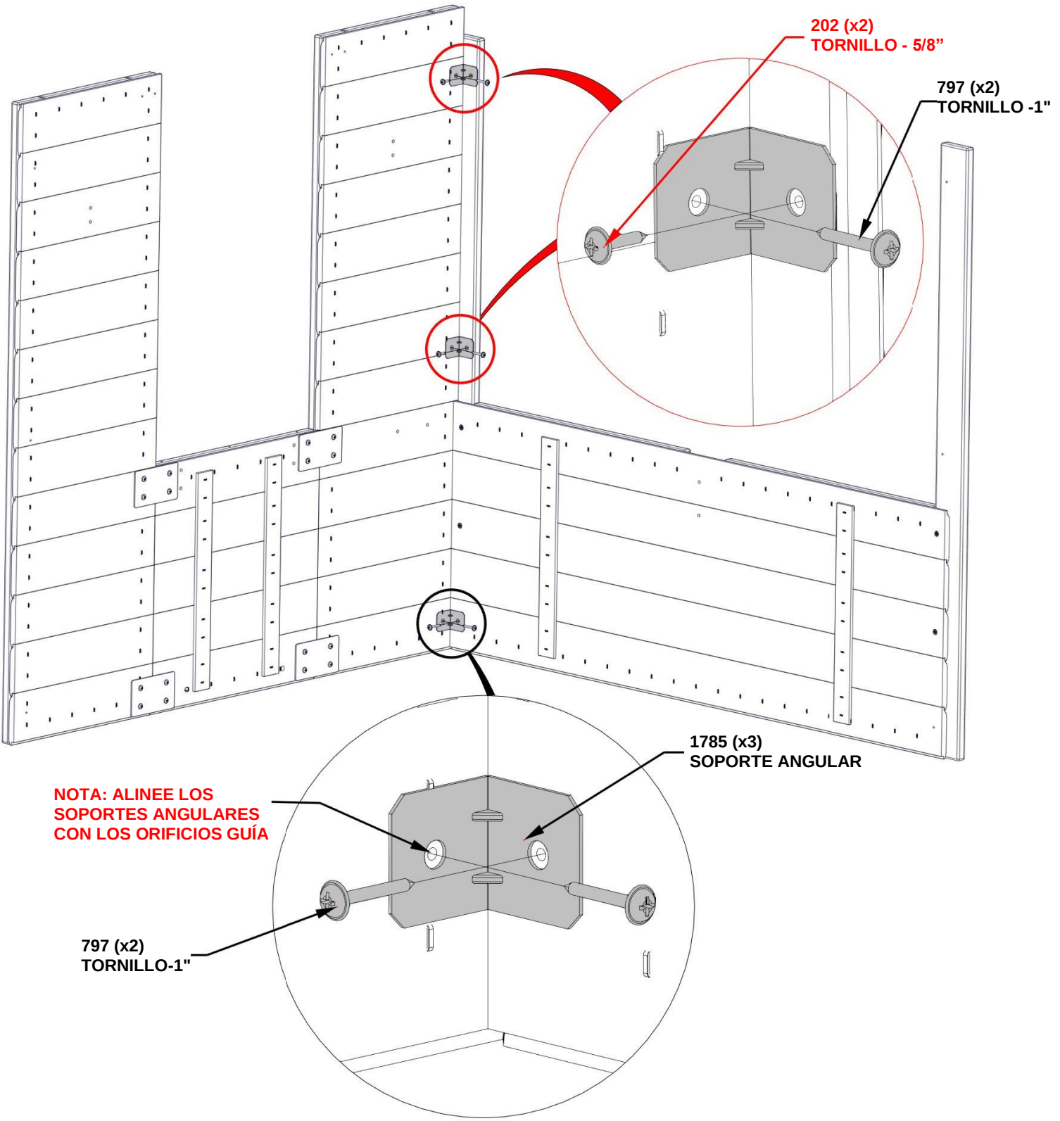
A4M01785 (x3) SOPORTE ANGULAR
