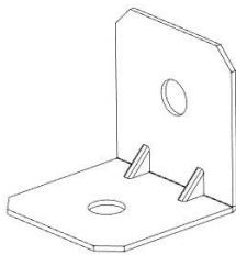
A4M01785 (x3) SOPORTE ANGULAR
