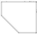
G3 SOPORTE DEL ESTANTE - W4L17342 (x1) 15/16"x5 1/4"x5 7/8" (24x134x150)
