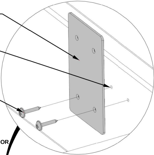
997(x2) LISTÓN DE METAL
