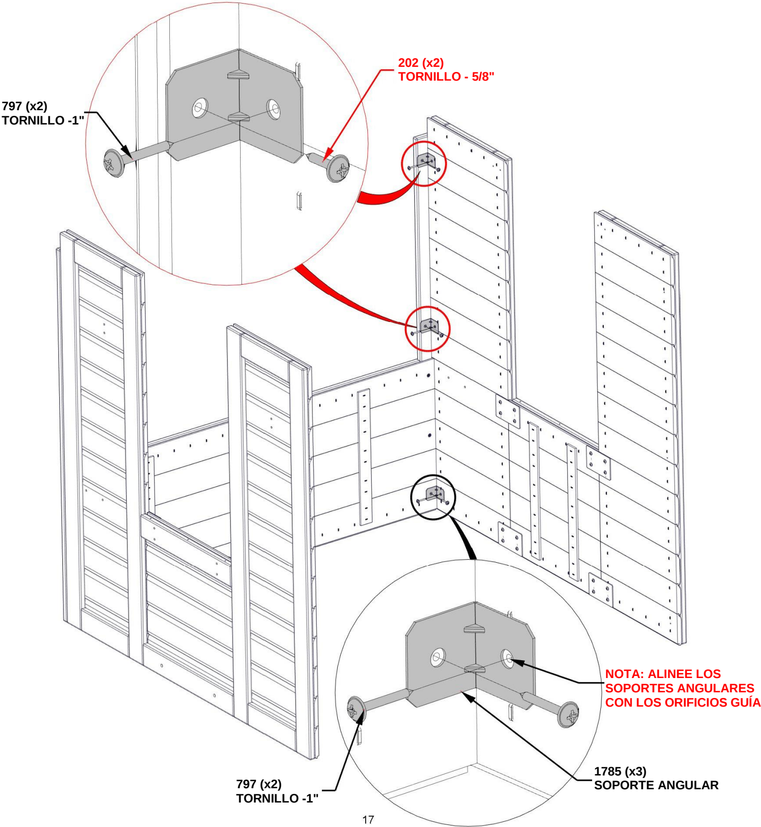
A4M01785 (x3) SOPORTE ANGULAR
