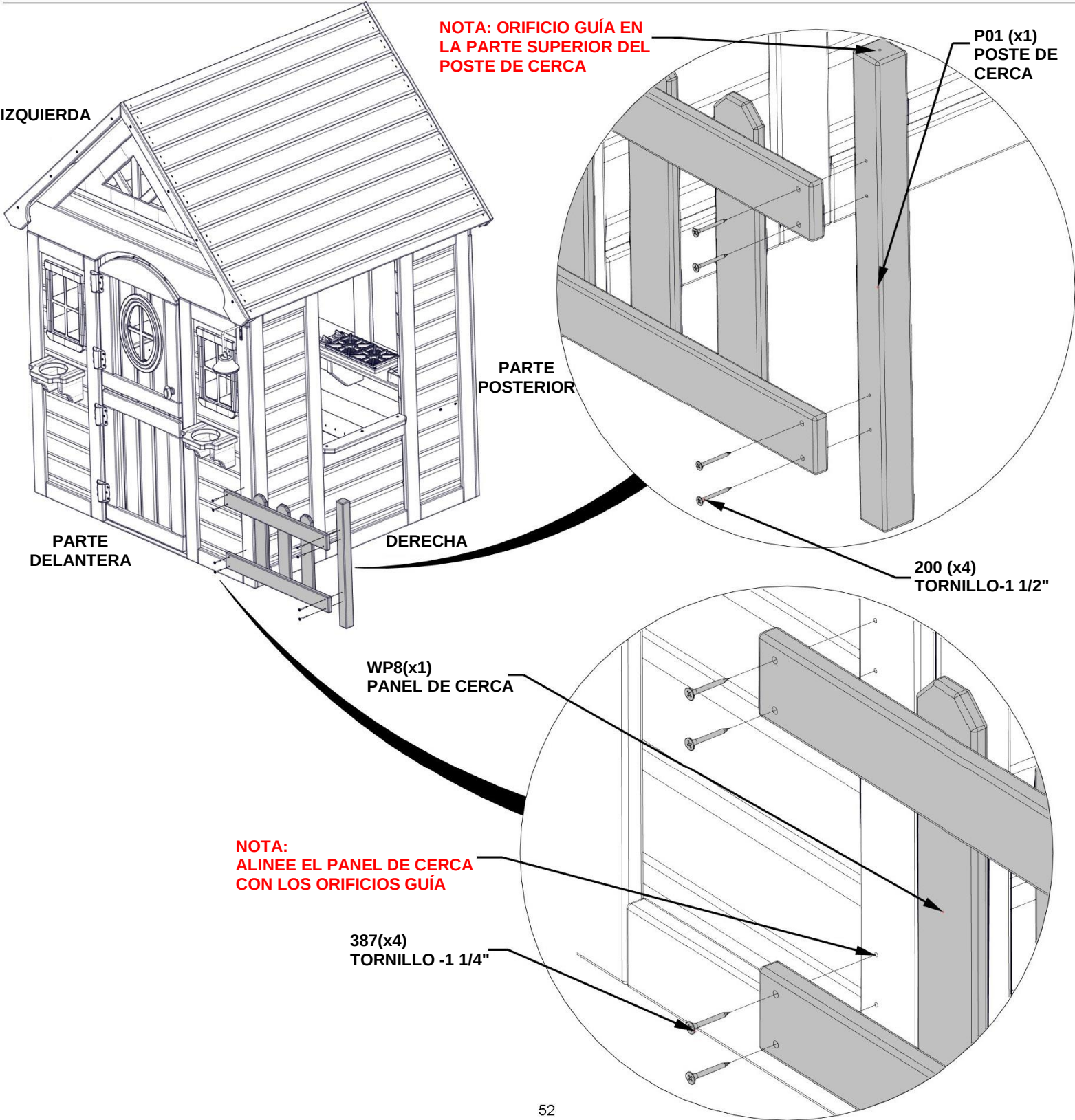
WP8 PANEL DE CERCA - W2A03584 (x1) 1 1/8"x13"x21 1/16" (28x330x535)
