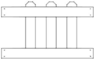
WP8 PANEL DE CERCA - W2A03584 (x1) 1 1/8"x13"x21 1/16" (28x330x535)
