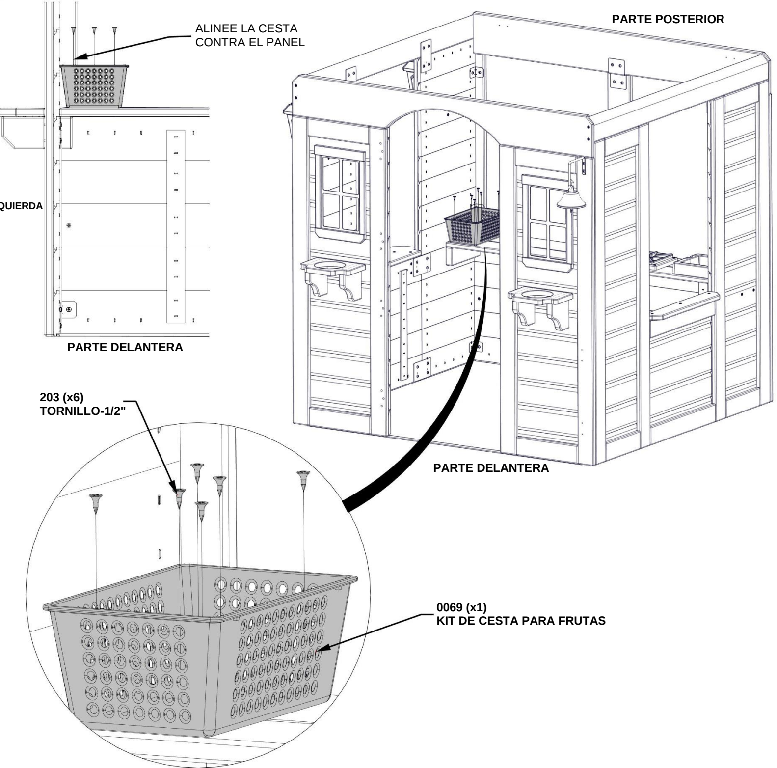
A6P00069 (x1) KIT DE CESTA PARA FRUTAS
