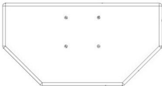
H4 SOPORTE DEL ASIENTO DEL BANCO - W4L17337 (x2) 15/16"x3 3/8"x6 9/16" (24x86x166)
