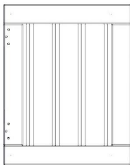
DP1 PANEL INFERIOR DE LA PUERTA - W2A03580 (x1) 1 1/16"x15 11/16"x19 11/16" (27x398x500)
