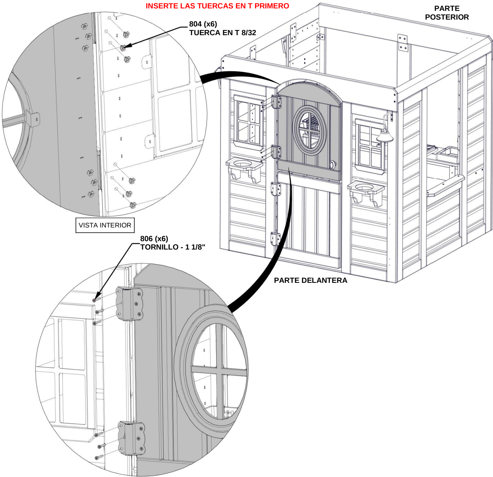
MONTAJE SUPERIOR DE LA PUERTA
