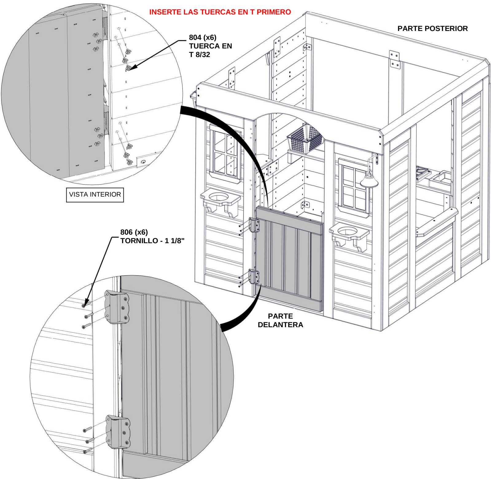
MONTAJE DE LA PUERTA INFERIOR
