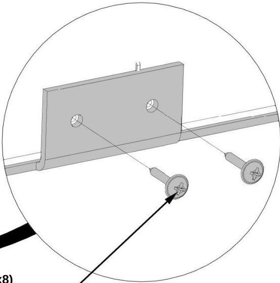
392 (x8) TORNILLO - 3/4"
