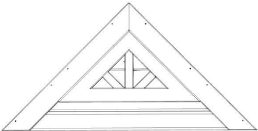
(x2) MONTAJE DEL PANEL DEL GABLETE DEL PASO ANTERIOR
