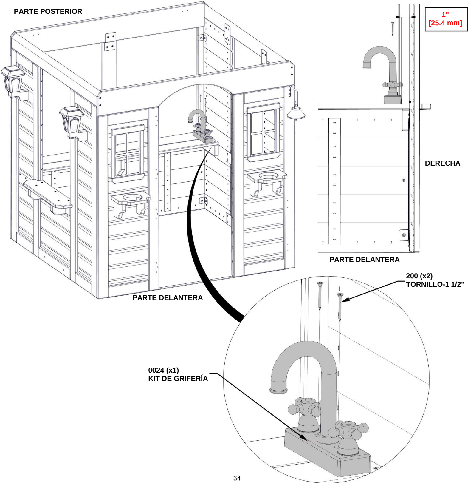
A6P00024 (x1) KIT DE GRIFERÍA
