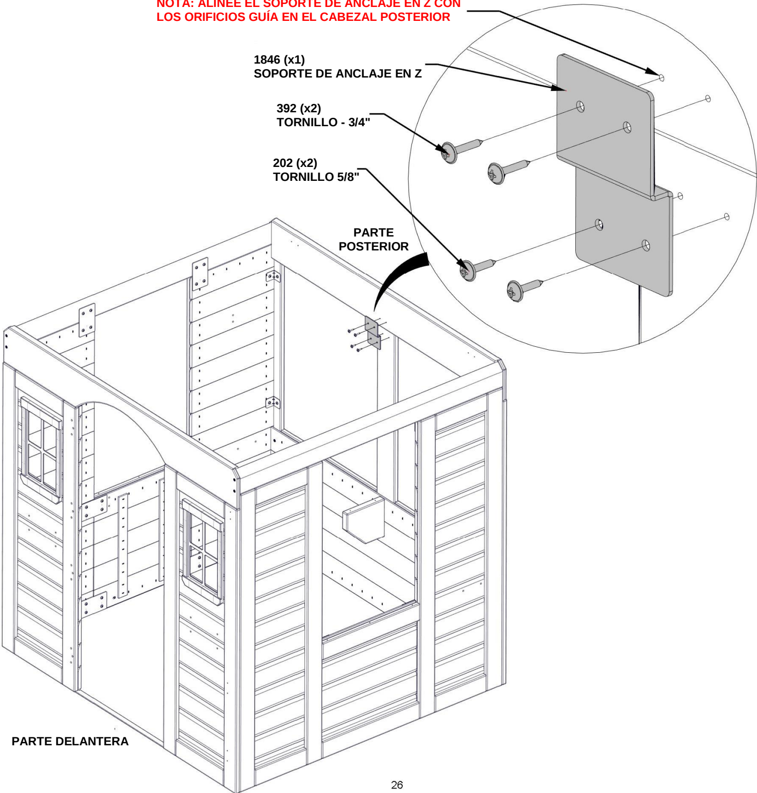
A4M01846 (x1) SOPORTE DE ANCLAJE EN Z
