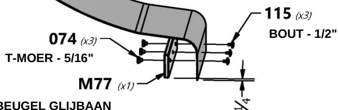
BEUGEL GLIJBAAN
